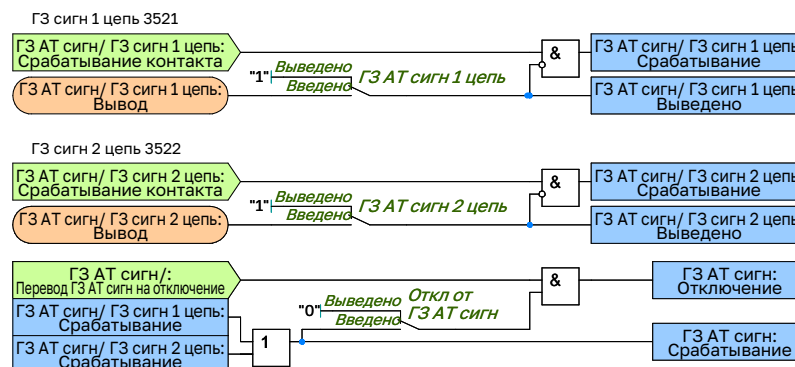
Рисунок 2.12 – Функциональная схема логики сигнальной ступени ГЗ
