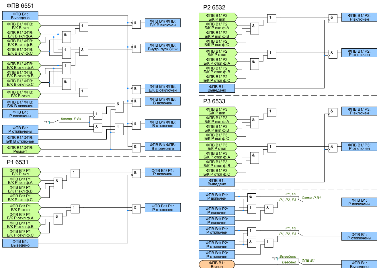
Рисунок 2.44 – Функциональная схема логики ФПВ В1(ЛВ) ВН
