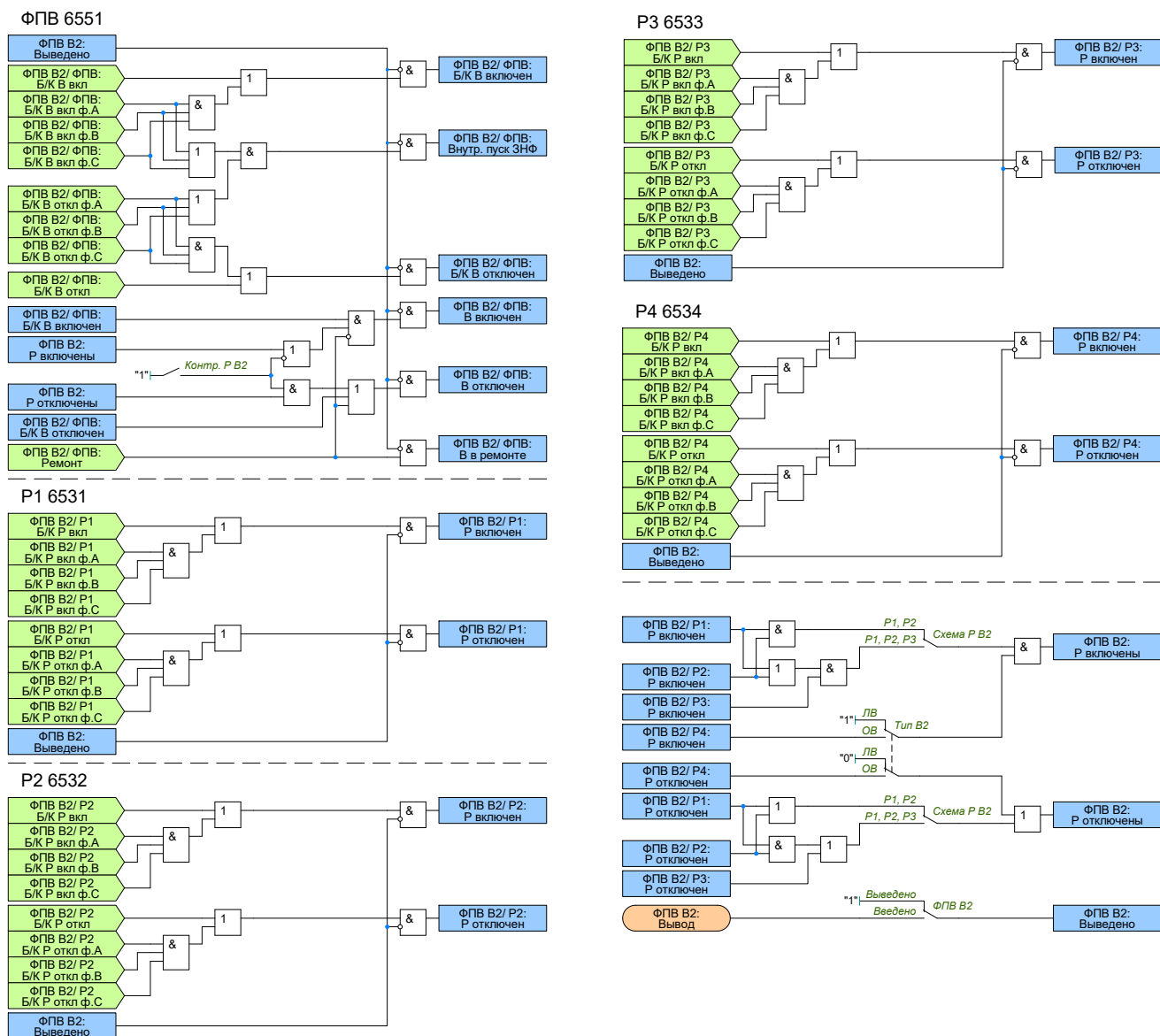
Рисунок 2.45 – Функциональная схема логики ФПВ В2(ОВ) ВН
