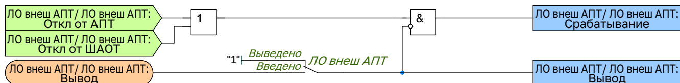
Рисунок 2.39 – Функциональная схема логики внешних отключений АПТ
